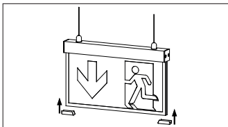
Abb. 5 Piktogramme mit den Halteklammern sichern.
