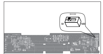
Abb. 8 M = Dauerschaltung NM = Bereitschaftsschaltung
