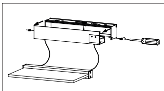
Abb. 1 Gehäuse an den seitlichen Vorkehrungen öffnen und Montageteil abnehmen.
