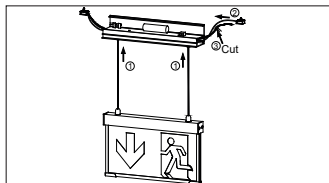
Abb. 6 1) Seilpendel auf die passende Länge einstellen 2) Seil aus der Klemme entnehmen 3) Seil kürzen und an der Klemme anschließen
