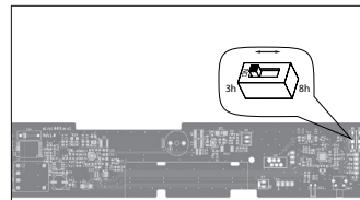
Abb. 7 Wahlweise 3 h oder 8 h Überbrückungszeit einstellbar.
