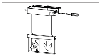
Abb. 10 Gehäuse auf Montageteil schieben und Gehäuse verschließen.
