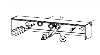
Abb. 3 Anschließend Schutzleiter anschließen. Beiliegenden Stecker anschließen.
