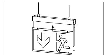
Abb. 4 Gewünschte Piktogramme an den Scheibenhalter aufstecken.
