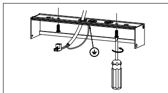
Abb. 2 Anschlusskabel einführen, Montageteil an der Decke oder an der Wand (Abb.3) befestigen.
