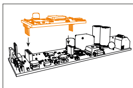
Abb. 3 Add-On aufstecken.
