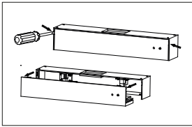
Abb. 1 Gehäuse öffnen.
