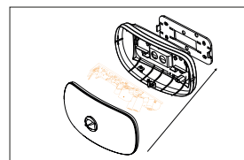
Abb. 5 Gehäuse schließen.
