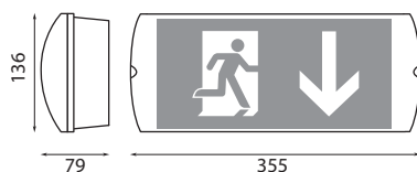
Maßzeichnung HA (alle Angaben in mm)
