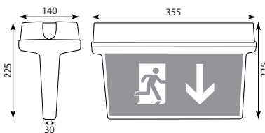
Maßzeichnung HA mit Haube (alle Angaben in mm)
