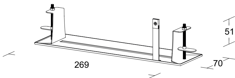
Maßzeichnung
