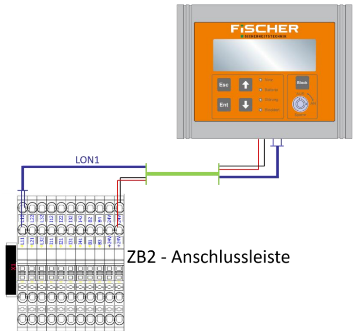
Abbildung 23 ZBX-FMS Anschluss
