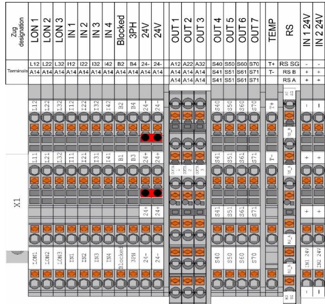
Abbildung 17 Steueranschlüsse
