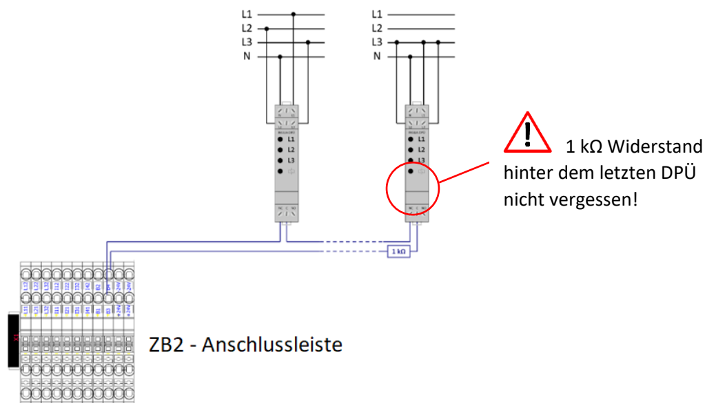
Abbildung 27 DPÜ Anschluss
