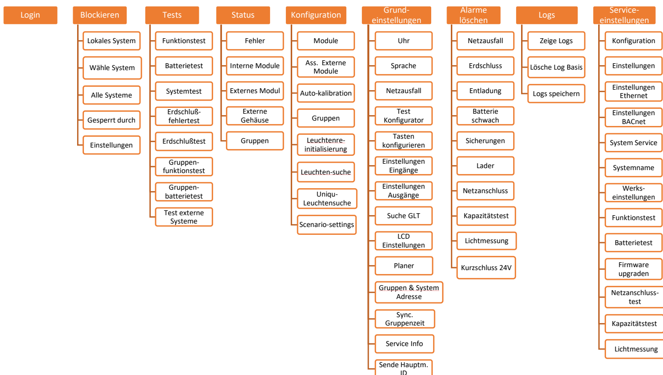
Abbildung 33 Menüstruktur
