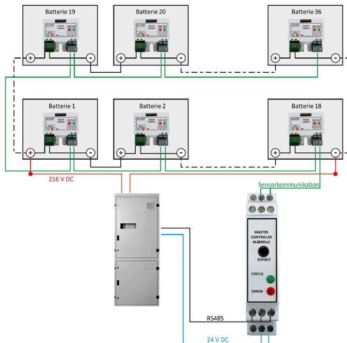
Abbildung 11 Anschlussplan IBMS
